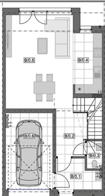
ZESTAWIENIE POWIERZCHNI - POZIOM 0
