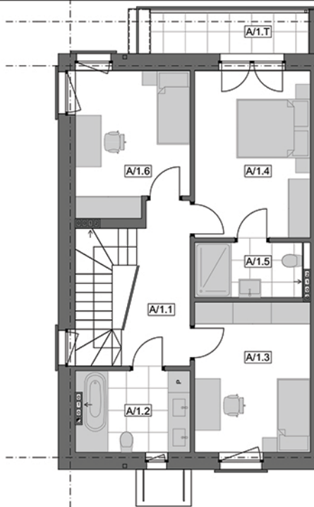
ZESTAWIENIE POWIERZCHNI - POZIOM +1
