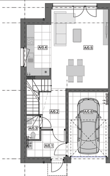
ZESTAWIENIE POWIERZCHNI - POZIOM 0
