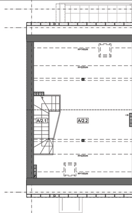
PODDASZE NIEUŻYTKOWE
