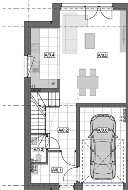
ZESTAWIENIE POWIERZCHNI - POZIOM 0
