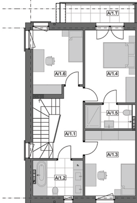
ZESTAWIENIE POWIERZCHNI - POZIOM +1
