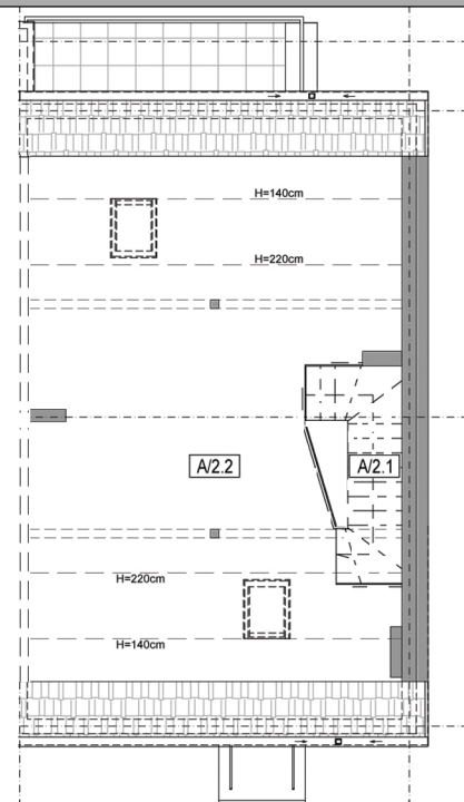
PODŁOŻE NIEUŻYTKOWE
