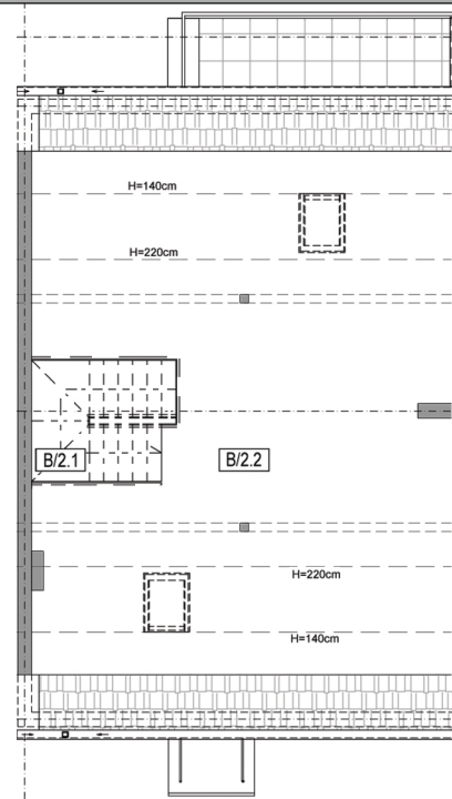
PODDASZE NIEUŻYTKOWE
