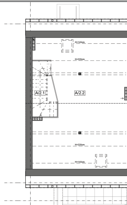
PODDASZE NIEUŻYTKOWE
